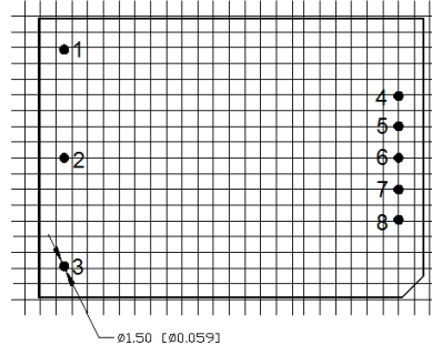
PCB 推荐图
